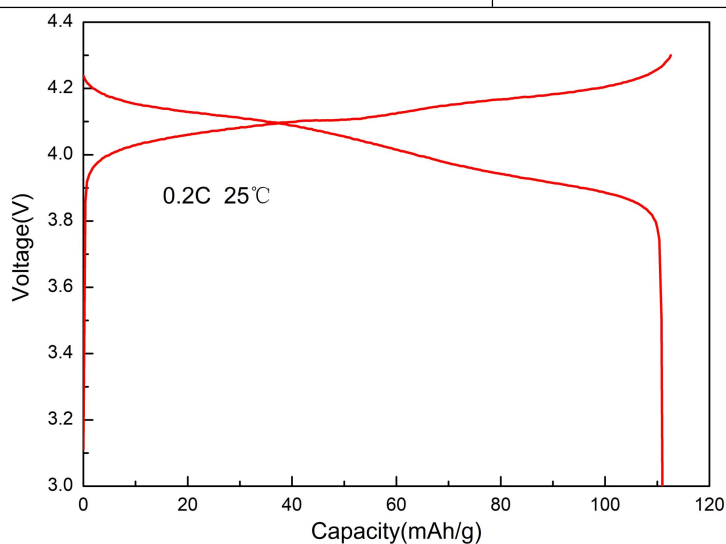
DXM-1182A 充放电曲线
