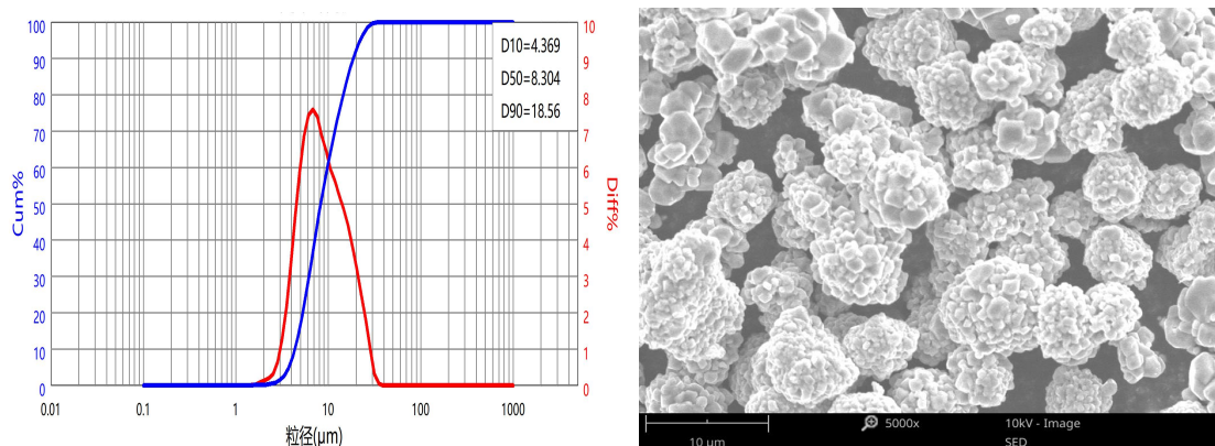
DXM-1182A 激光粒度分布曲线
