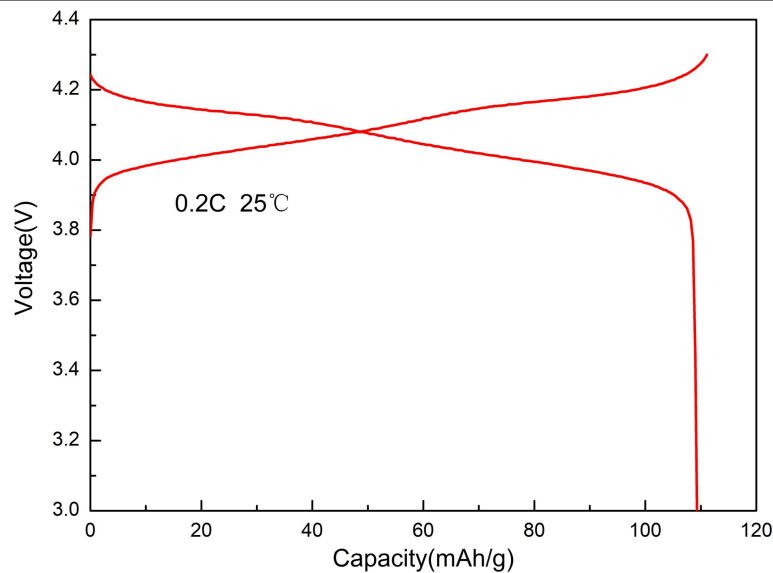
DXM—2000 充放电曲线
