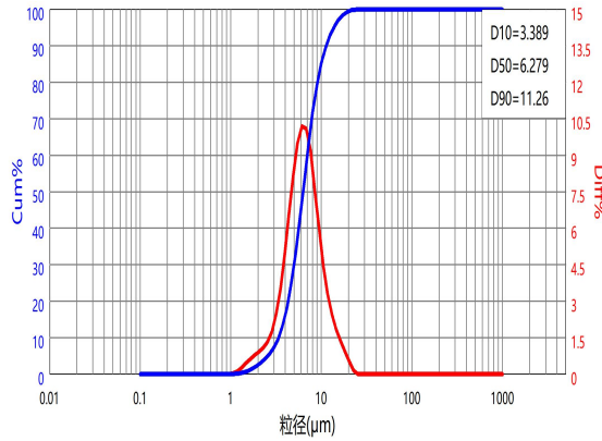
DXM—2000 激光粒度分布曲线
