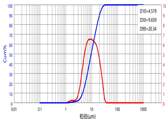
DXM-1000 激光粒度分布曲线
