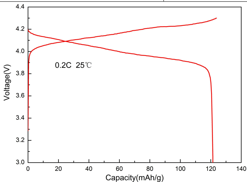
DXM-1000 充放电曲线
